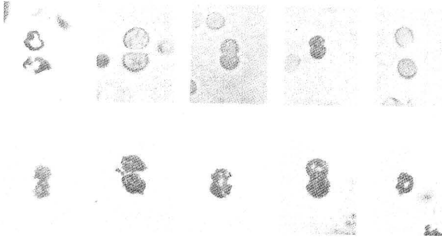
Fig. 12. A la izquierda: Fotografía de fósiles de lo que se presume fueron bacterias encontradas en depósitos de más de tres mil millones de años. A la derecha: Fotografías de bacterias vivientes actuales, cuya forma es comparable a la de los fósiles reproducidos a la izquierda.
