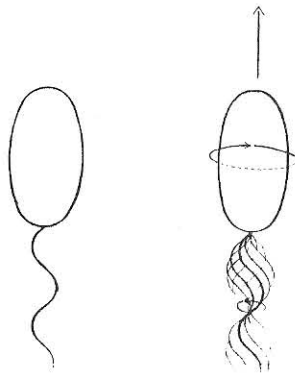
Fig. 42. Propulsión flagelar en la bacteria.
